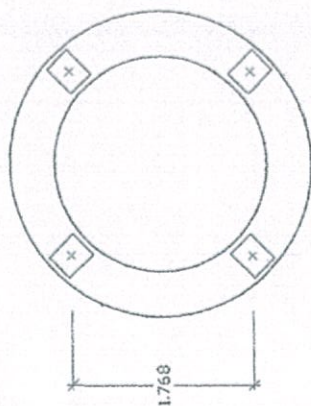
แปลนฐานโค้งก้นถัง 1:50
