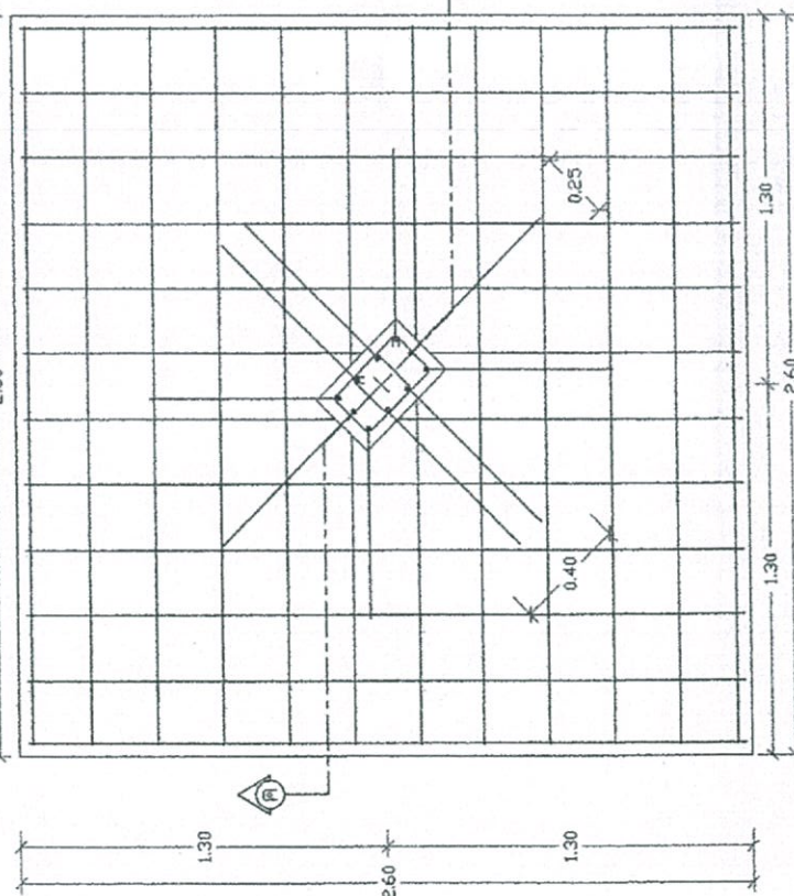
แปลงสุพรรณภูมิ แบบไม่ดอกเสี้ยว F1 1:20
