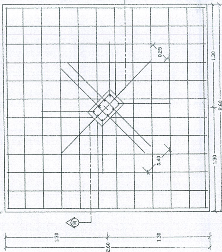
แปลงสุพรรณภูมิ แบบไม่ตอกเสาเข็ม F1 1:20
